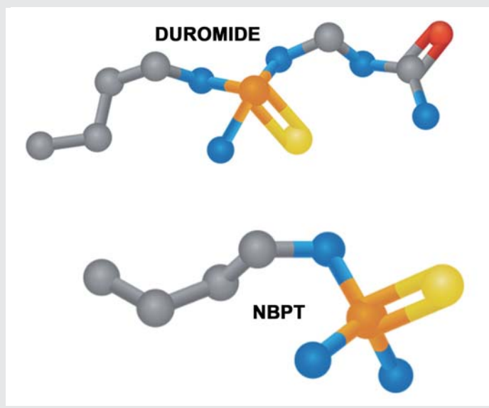
Figuur 1: Duromide en NBPT is twee aktiewe bestanddele in Kynoplus Pro®.
